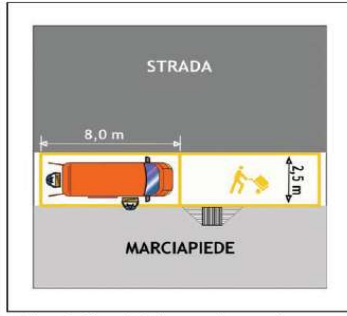
Figura 2 - Piazzola in linea con la carreggiata
